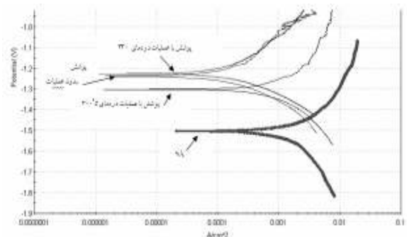
شکل ۵. منحنی پلاریزاسیون تافل پایه منیزیمی و پوشش با عملیات حرارتی
