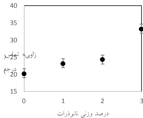
شکل ۴. منحنی زاویه تماس قطره آب بر روی نمونه‌های نانوکامپوزیتی برحسب درصد نانوسیلیکا.
