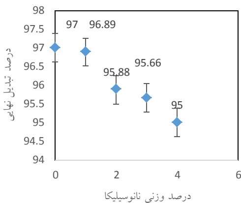
شکل ۱ درصد تبدیل نمونه‌های نانوکامپوزیتی بر حسب درصد وزنی نانوذرات سیلیکای موجود در نمونه‌ها.
