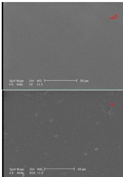
شکل ۵. تصاویر میکروسکوپ الکترونی روبشی از سطح شکست نمونه شاهد (بالایی) و نمونه حاوی ۲٪ نانوذرات سیلیکا (پایینی).
