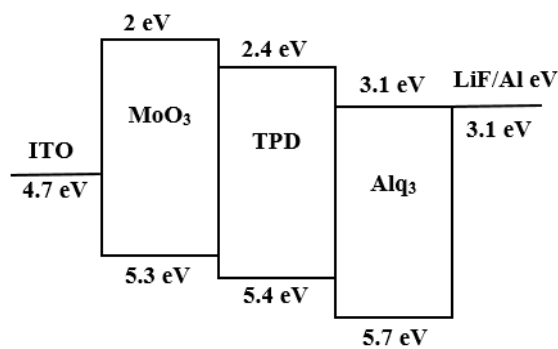
شکل ۲: نمودار ترازهای انرژی برای ساختار دیود نورگسیل آلی
