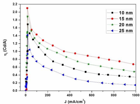
شکل ۹. نمودار بازده جریان بر حسب چگالی جریان برای دیودهای ساخته شده با ضخامت‌های متفاوت لایه \text{MoO}_3
