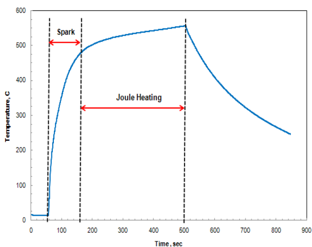
شکل ۱. تغییرات دما بر حسب زمان را در حین تف‌جوشی پودر آلومینیم-گرافیت بوسیله SPS
