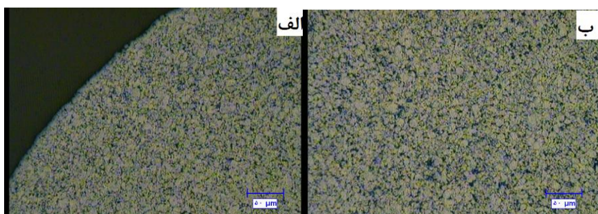
شکل ۳. الف-تصویر OM کامپوزیت Al – 3% Gr ب- تصویر OM کامپوزیت Al – 4.5% Gr (به روش همگن‌شده در مایع-SPS).
