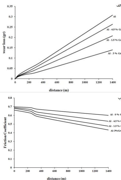
شکل ۸ الف- نمودار سایش و ب- ضریب اصطکاک: کامپوزیت Al-Gr با درصدهای مختلف گرافیت و آلومینیم خالص تولید شده به روش همگن سازی در فاز مایع و SPS در فشار ۲۸ MPa.
