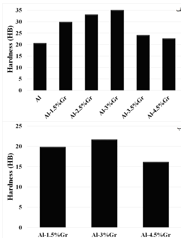
شکل ۶. الف- نمودار سختی کامپوزیت Al-Gr با درصد‌های مختلف گرافیت تولید شده به روش همگن سازی در فاز مایع و SPS در فشار ۲۸ MPa و ب- نمودار سختی کامپوزیت Al-Gr با درصد‌های مختلف گرافیت تولید شده به روش همگن سازی در فاز مایع و SPS در فشار ۱۴ MPa.
