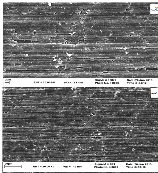
شکل ۱۱. الف و ب- تصاویر میکروسکوپ الکترونی روبشی (SEM) تهیه شده از سطح سایش ۱-۱.۵٪Gr
