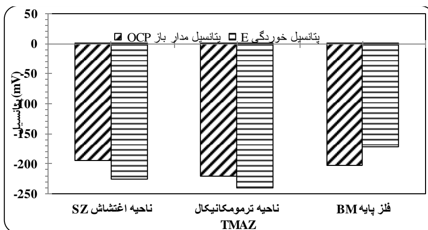
شکل ۸. پتانسیل مدار باز (OCP) و پتانسیل خوردگی (E) در نواحی مختلف جوش.
