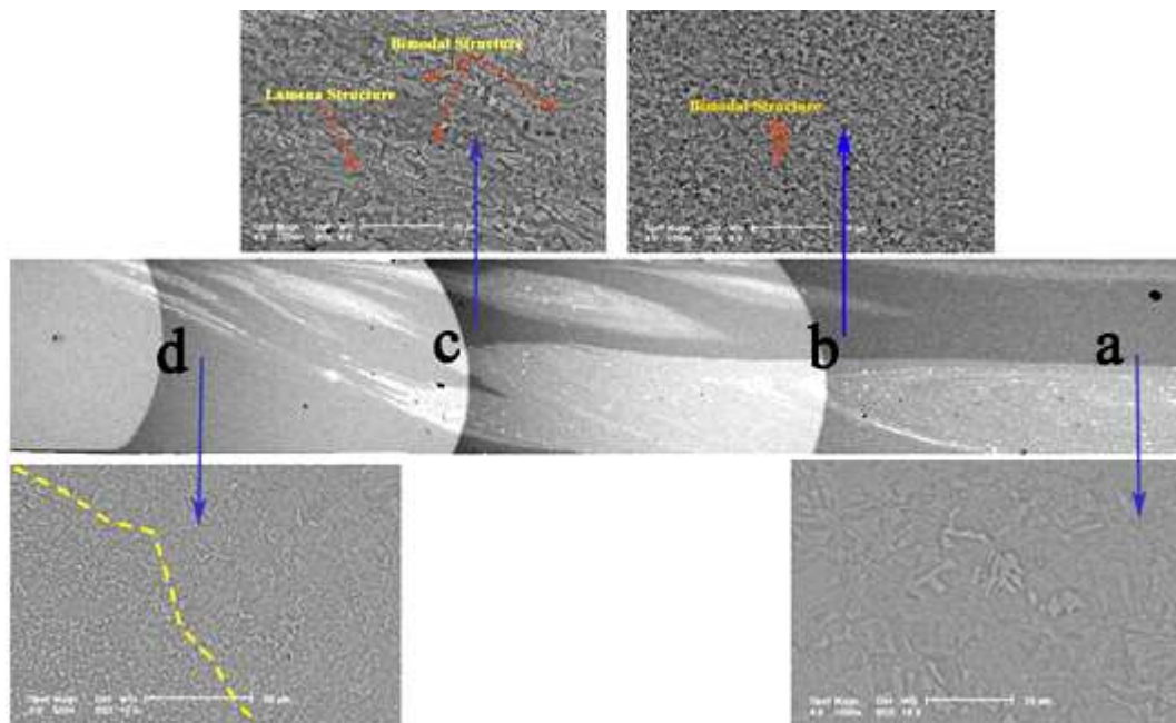
شکل ۳. تصویر میکروسکوپی الکترونی روبشی از ریز ساختار نواحی مختلف جوش a: ناحیه اغتشاش، b تا c: ناحیه انتقال و d: فلز پایه.
