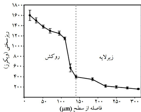
شکل ۱۰. تغییرات میانگین ریزسختی در روکش و زیرلایه فولادی.
