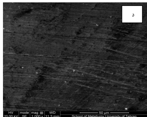
شکل ۸. الف) نمودار ضریب اصطکاک پوشش Co-۵/۶P قبل از عملیات حرارتی و ب) بعد از عملیات حرارتی، ج) تصویر میکروسکوپ الکترونی از سطح سایش پوشش Co-۵/۶P قبل از عملیات حرارتی و د) بعد از عملیات حرارتی.
