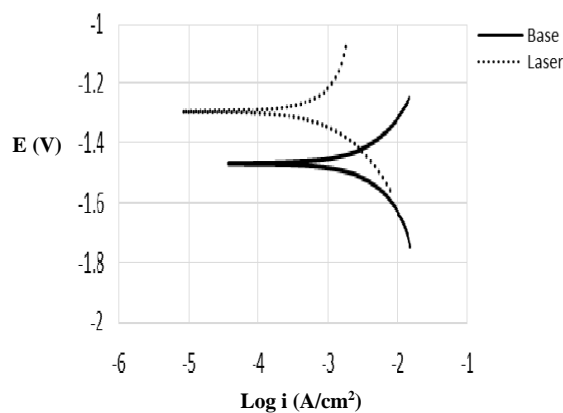
شکل ۵. منحنی‌های پلاریزاسیون تافل آلیاژ پایه و نمونه تحت عملیات لیزر در محلول 3/5 درصد کلرید سدیم.
