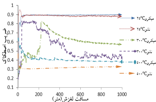
شکل ۵. نمودارهای ضریب اصطکاک برحسب مسافت لغزش برای پوشش های میکرو و نانو ساختار Cr 2 O 3 در دمای محیط، ۳۰۰ و ۵۰۰ °C
