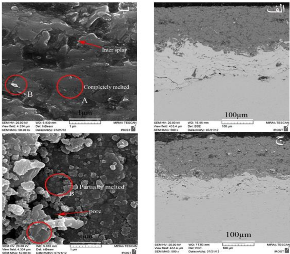
شکل ۲. تصاویر میکروسکوپی الکترونی (FE-SEM) از مقطع عرضی پوشش‌های \text{Cr}_2\text{O}_3 (الف و ب) پوشش میکروساختار (ج و د) پوشش نانو ساختار.
