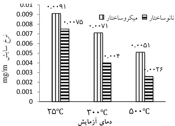
شکل ۴. نمودارهای نرخ سایش برای پوشش های Cr 2 O 3 در دمای محیط، ۳۰۰ °C و ۵۰۰ °C.
