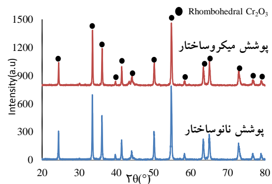
شکل ۱. الگوی پراش سنجی پرتو ایکس پوشش‌های \text{Cr}_2\text{O}_3 .
