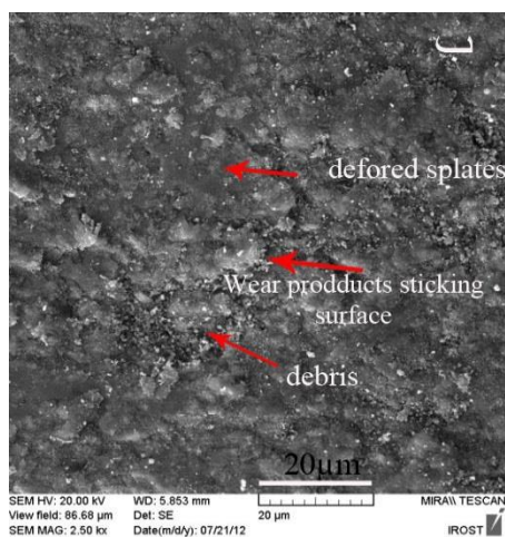
شکل ۶. تصاویر FE-SEM از سطح سایش پوشش های Cr_2O_3 توسط پین آلومینا در دمای محیط. (الف) پوشش میکروساختار (ب) پوشش نانو ساختار.
