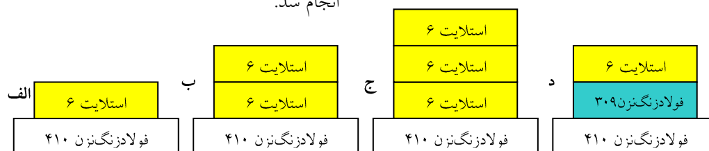
شکل ۱. شماتیک رویه سختی الف-۱ پاس ب-۲ پاس ج-۳ پاس د-بلا لایه میانی
