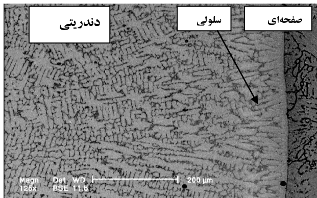
شکل ۵. تصویر میکروسکوپ الکترونی استلایت
