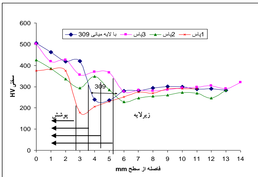
شکل ۱۱. نمودار سختی نمونه‌های ۱، ۲ و ۳ پاس و با لایه میانی
