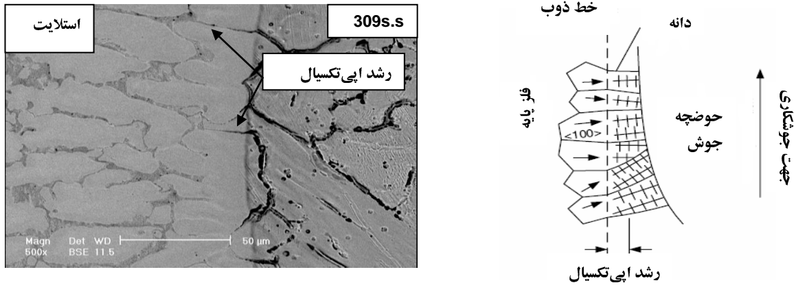
شکل ۸. تصویر میکروسکوپ الکترونی رشد اپی تکسیال در مرز استلایت ولایه
